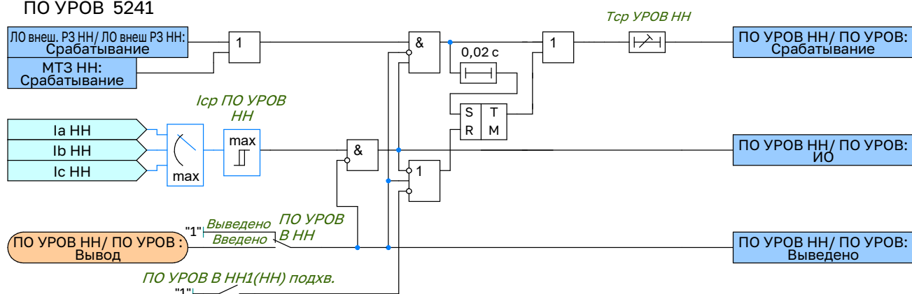
Рисунок 2.25 – Функциональная схема логики ПО УРОВ НН
